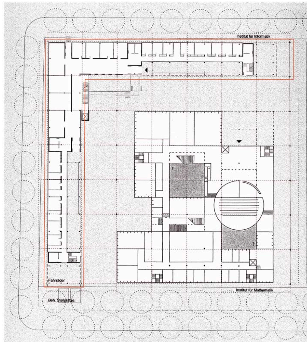
Grundriss beide Institute 1/800
